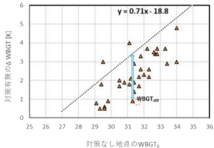
図4 実在するクールスポットにおける WBGT_0 、 \Delta WBGT 、および評価基準となる回帰式の例
