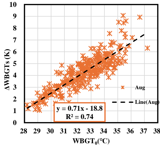
図3 近隣の気象台データを元で作成した完全日陰クールスポットの \Delta WBGT_s の回帰式
