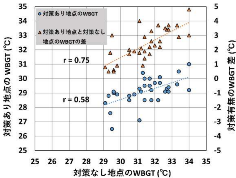
図1 対策なし地点と対策あり地点の相関関係
